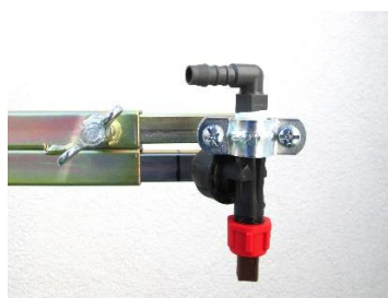
Düsenhalter Einstellung 90°
