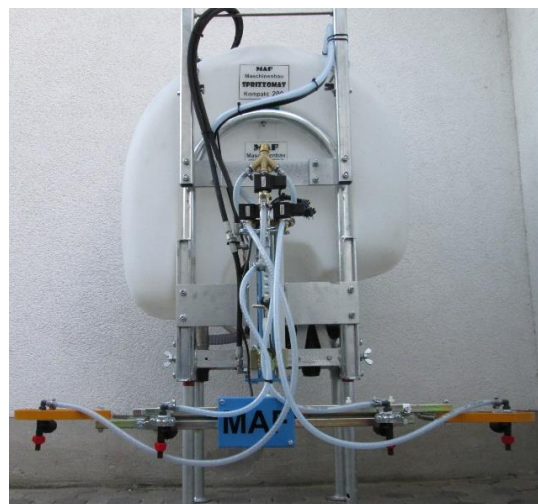
Ausstattung mit Bandspritzgestänge MAF uni 1 ED5m und hydraulischer Höhenverstellung und Ganzflächenabspritzung
