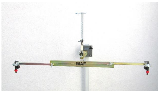
MAF uni 0sp 2/3 Düsenabstandsweite
