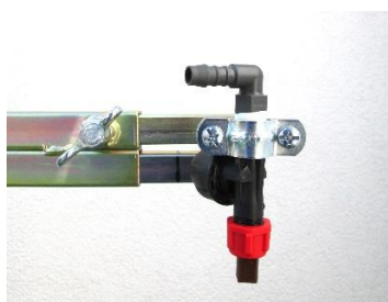
Düsenhalter Einstellung 90°
