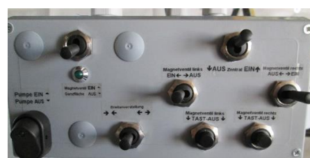
Elektrische Ansteuerung Typ 4 für Spritze mit Gestänge
