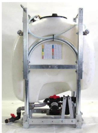
Ansicht Rückseite
