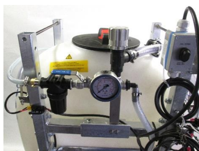
Druckregleinheit mit Steuerung
