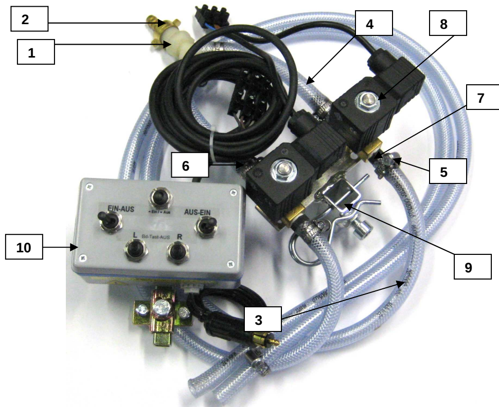
Abbildung Elektrische Düsenschialtung EDS01t1m
