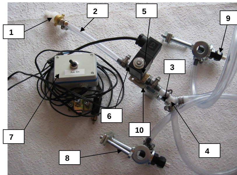
Abbildung Elektrische Düsenschialtung EDS01t1gf
